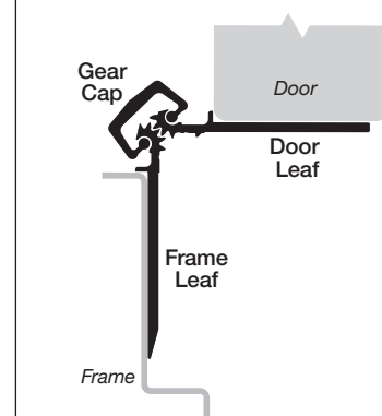
Fig. 2 Door Open 90°
