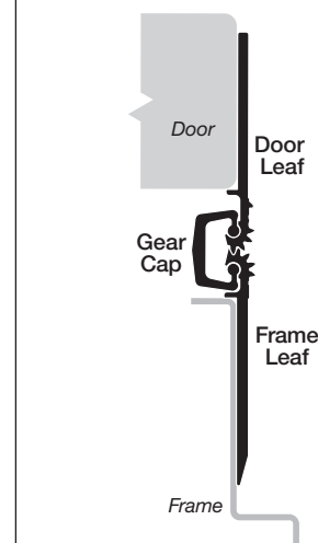
Fig. 3 Door Open 180°
