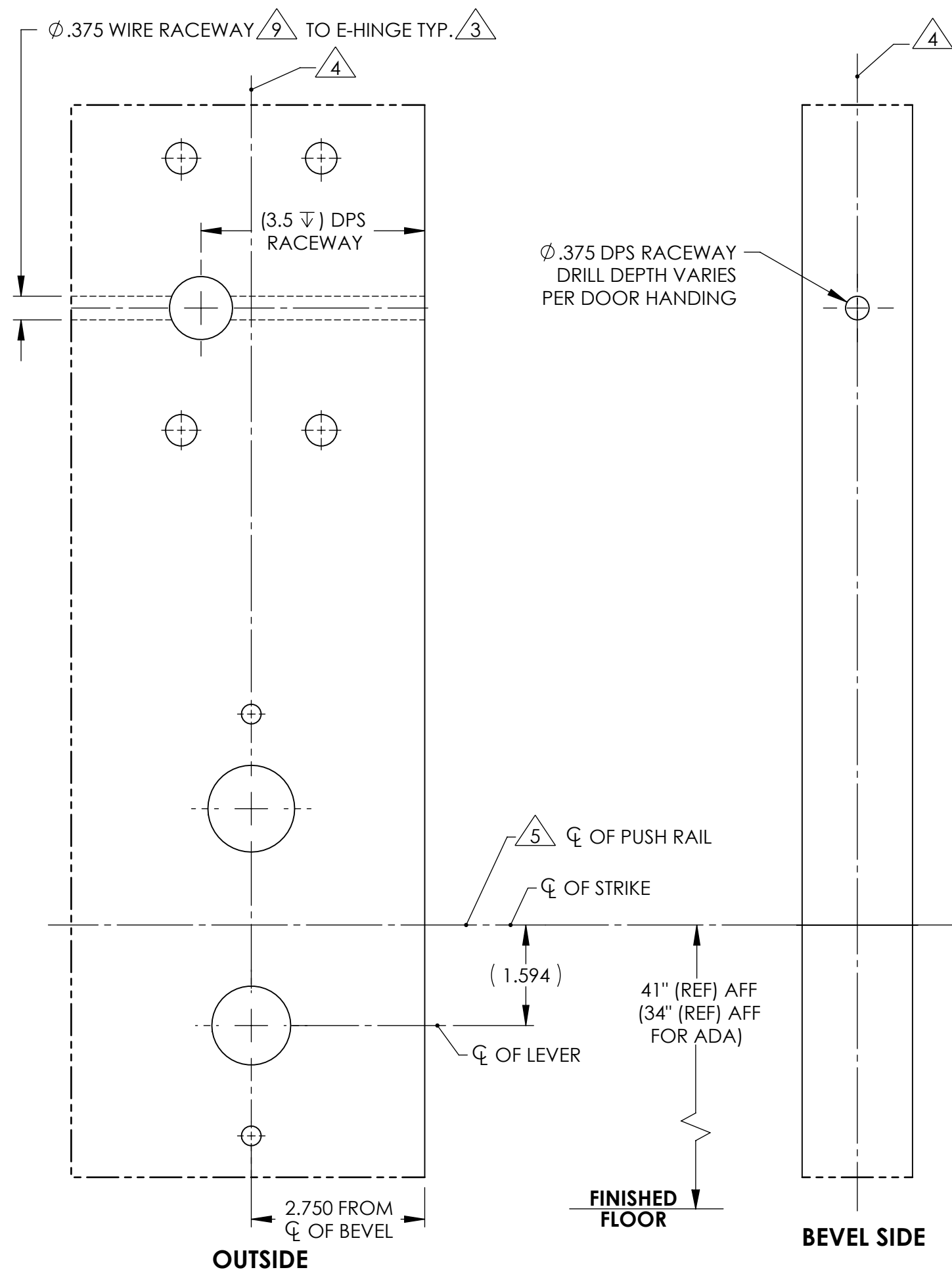
L.H.R.B. DOOR
