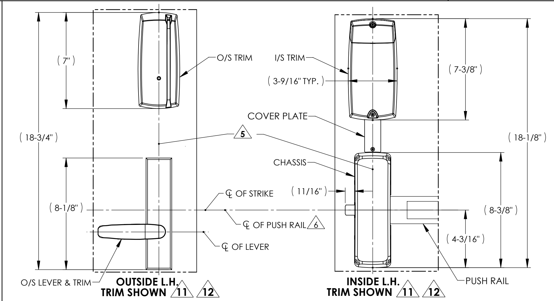
L.H.R.B. DOOR
