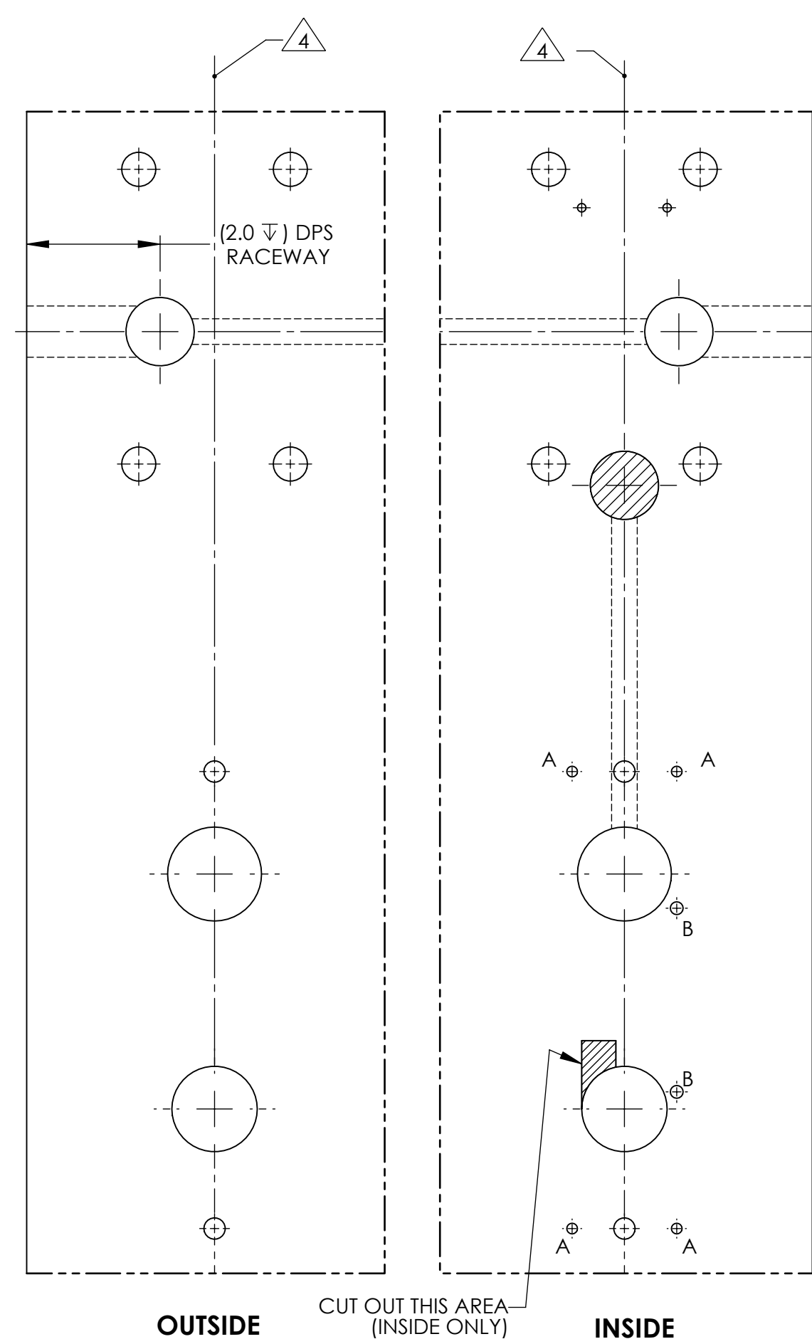
R.H.R.B. DOOR
