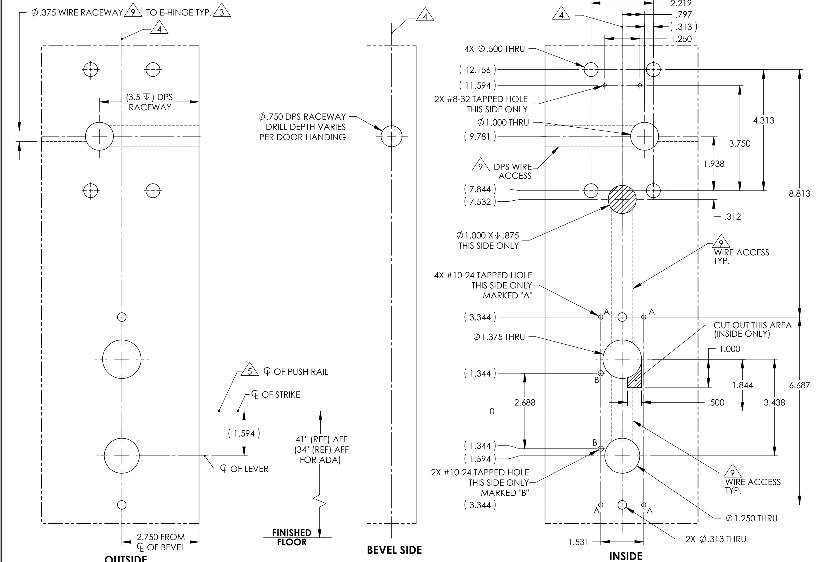
L.H.R.B. DOOR
