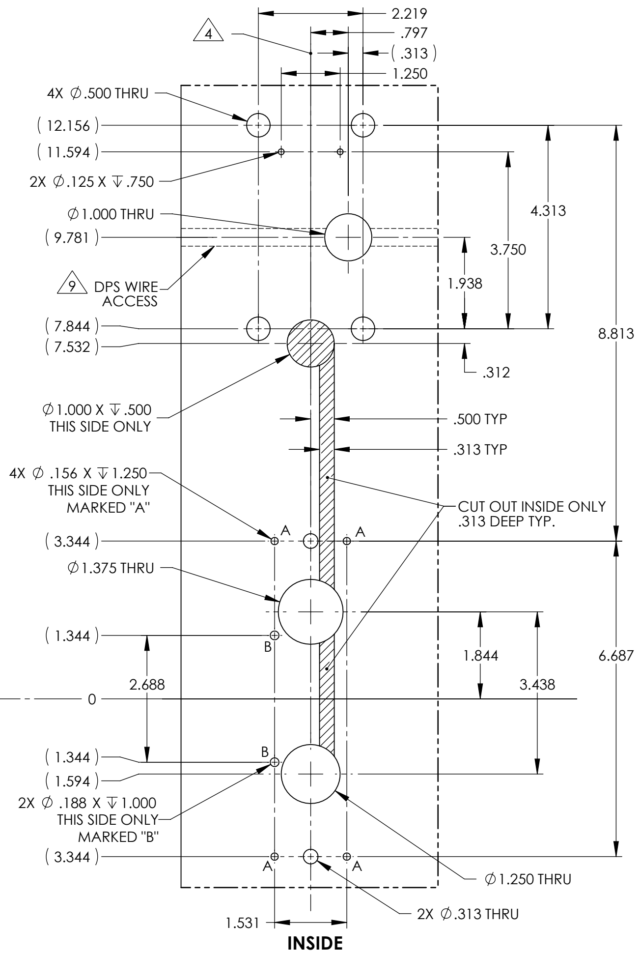
L.H.R.B. DOOR
